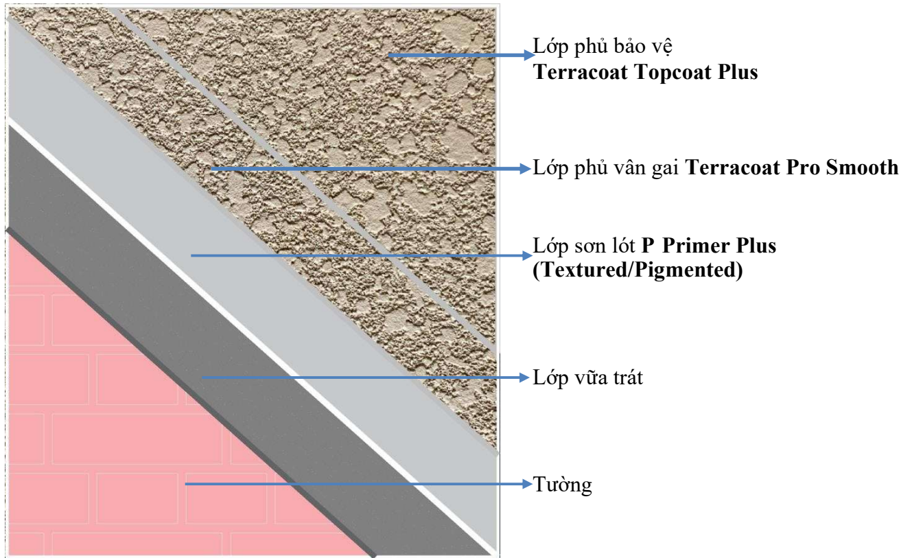
Hình 2. Cấu tạo hệ thống lớp phủ vân gai Terracoat Pro Smooth
